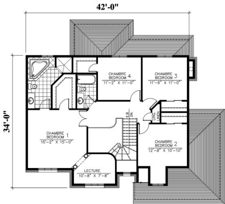
ÉTAGE : 1325 p.c. SECOND FLOOR : 1325 sq.ft.
