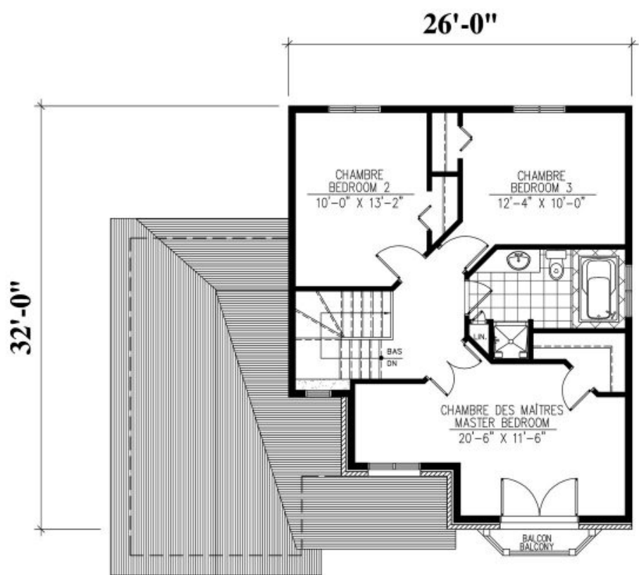
ÉTAGE : 760 p.c. SECOND FLOOR : 760 sq.ft.
