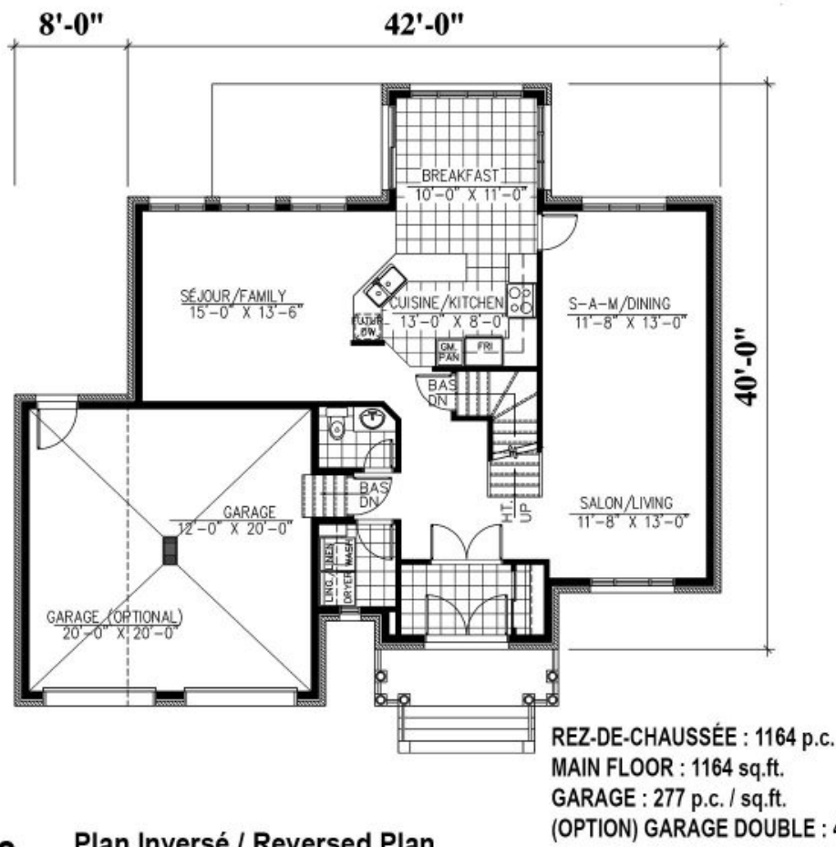
# 452 - Le Médoc Plan Inversé / Reversed Plan
