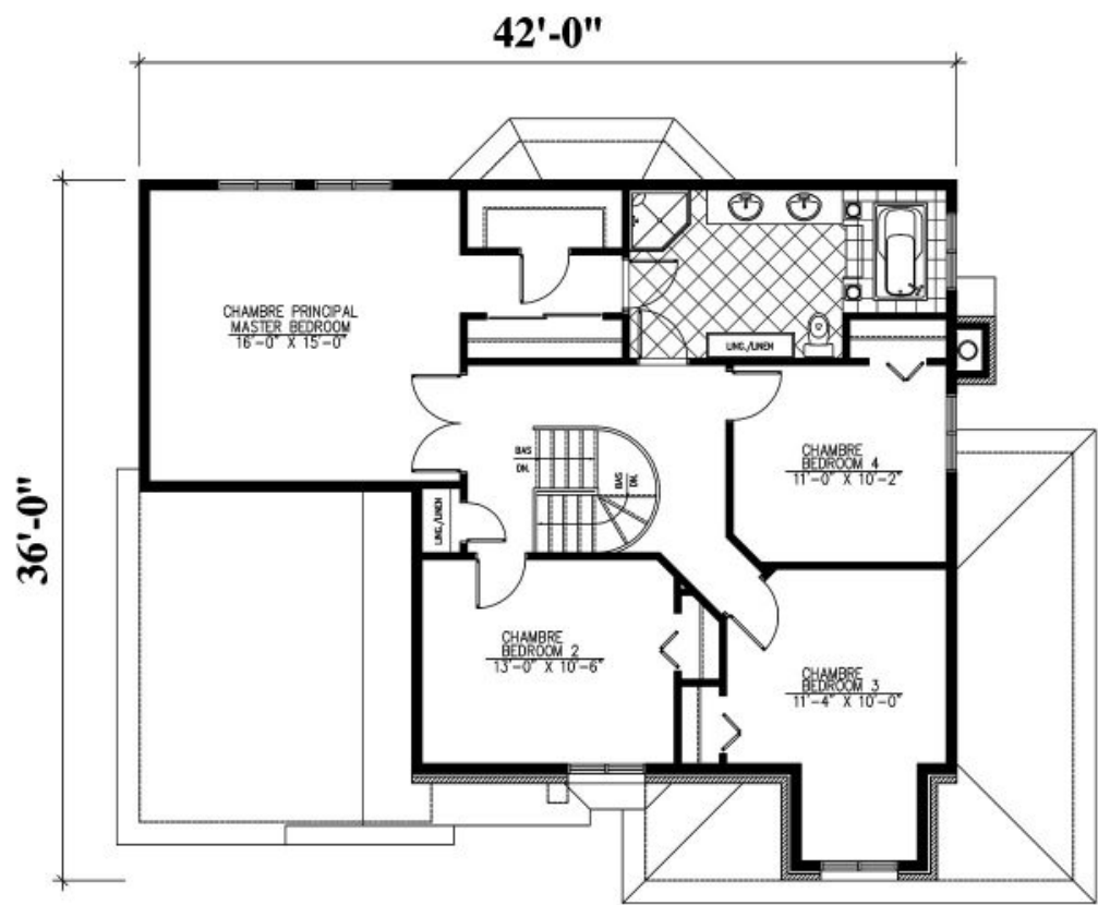
ÉTAGE : 1132 p.c. SECOND FLOOR : 1132 sq.ft.
