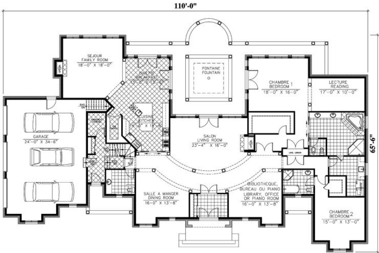
Plan Inversé / Reversed Plan # 474 - Le Gauvain
