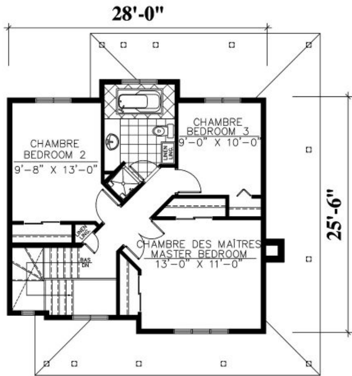
ÉTAGE : 708 p.c. SECOND FLOOR : 708 sq.ft.
