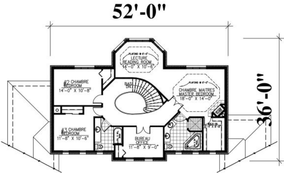
ÉTAGE : 1496 p.c. SECOND FLOOR : 1496 sq.ft.
