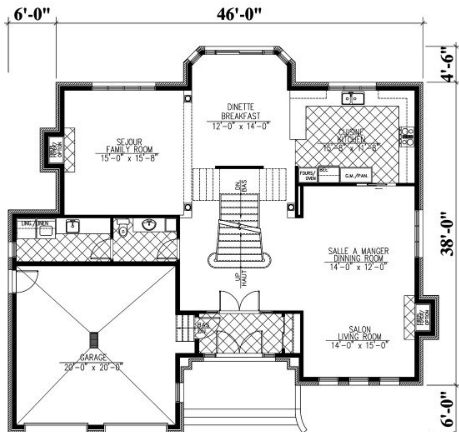
# 564 - Le Mimosa Plan Inversé / Reversed Plan
