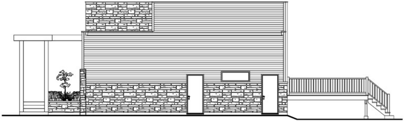
Latérale Droite
