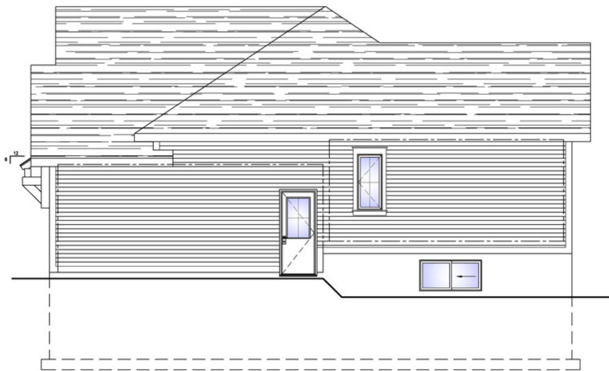
ÉLEVATION DROITE
