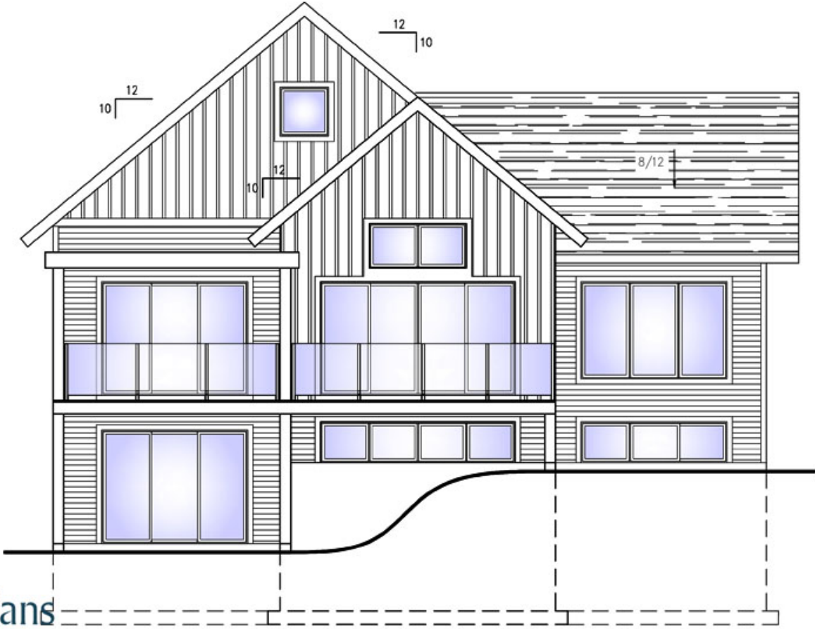
ÉLEVATION ARRIÈRE (VUE)
