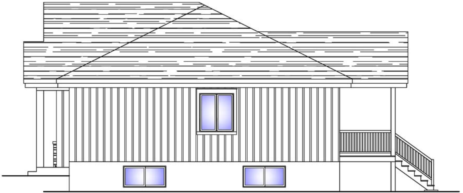
ÉLEVATION DROITE
