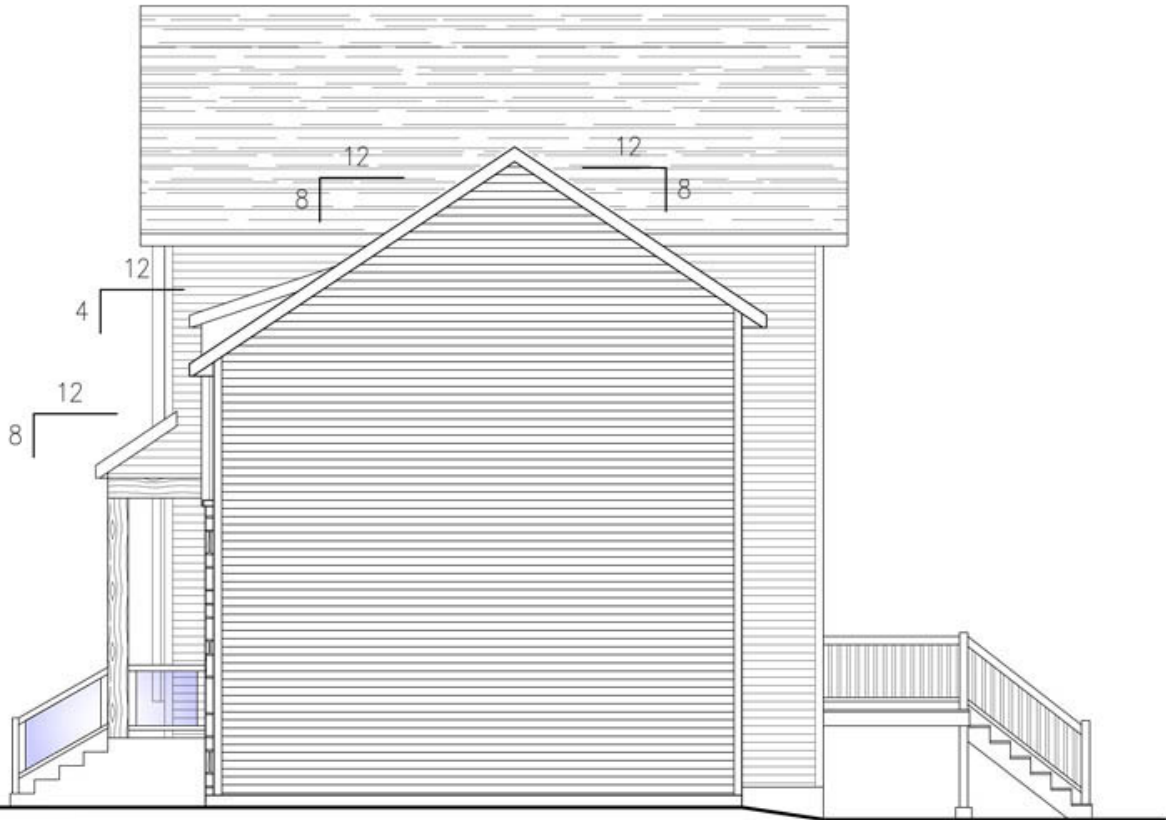
ÉLÉVATION DROITE
