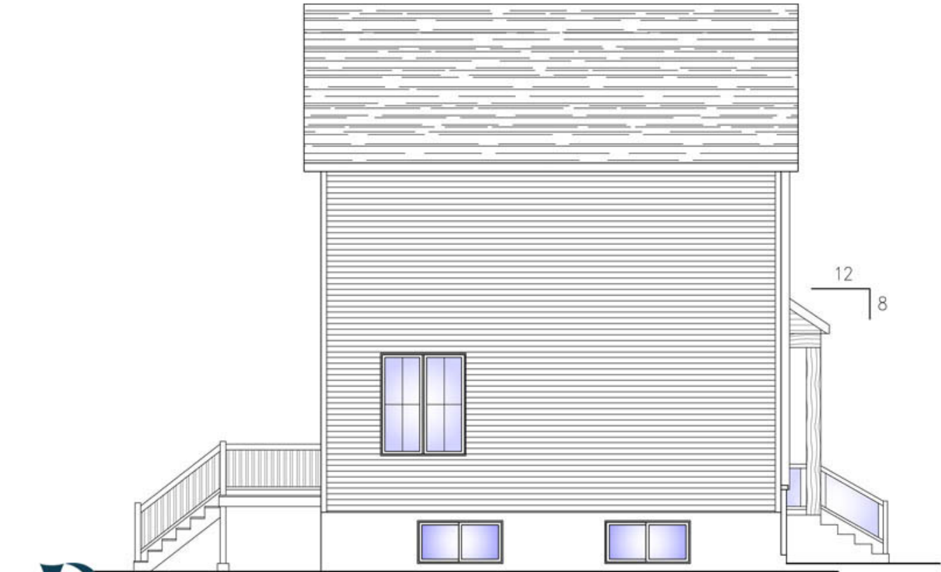
ÉLÉVATION GAUCHE
