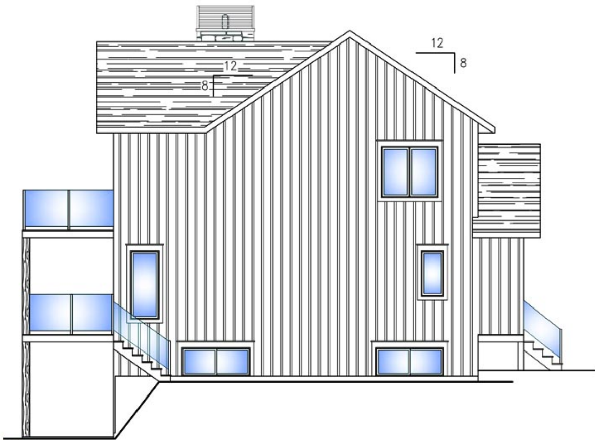
ÉLEVATION GAUCHE
