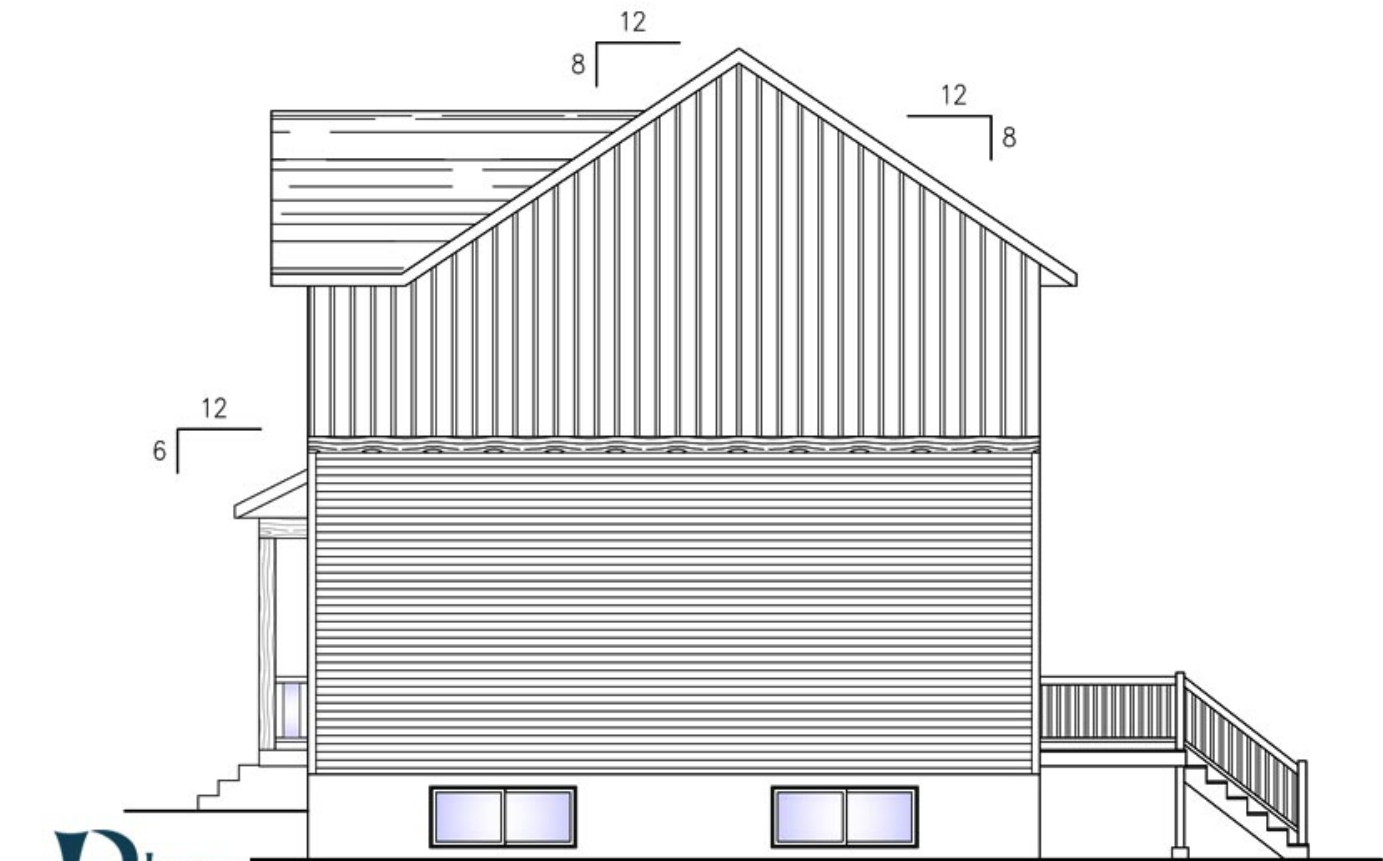
ÉLEVATION DROITE
