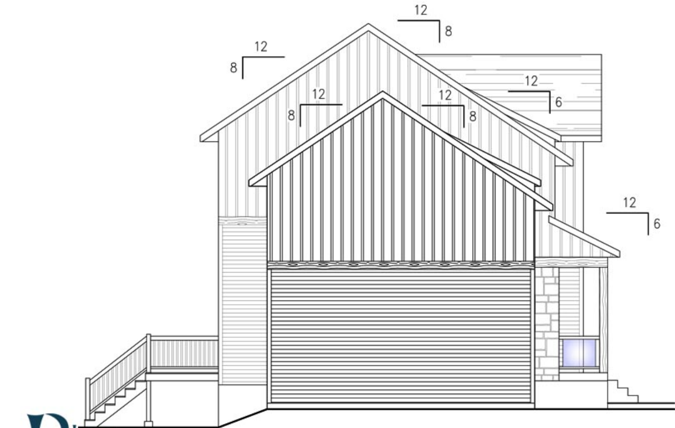
ÉLEVATION GAUCHE
