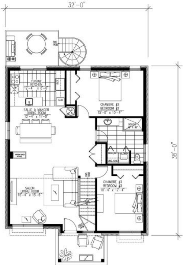
ÉTAGE : 1198 p.c. SECOND FLOOR : 1198 sq.ft.
