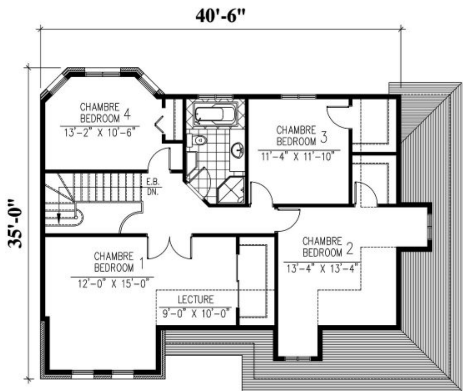
ÉTAGE : 1222 p.c. SECOND FLOOR : 1222 sq.ft.
