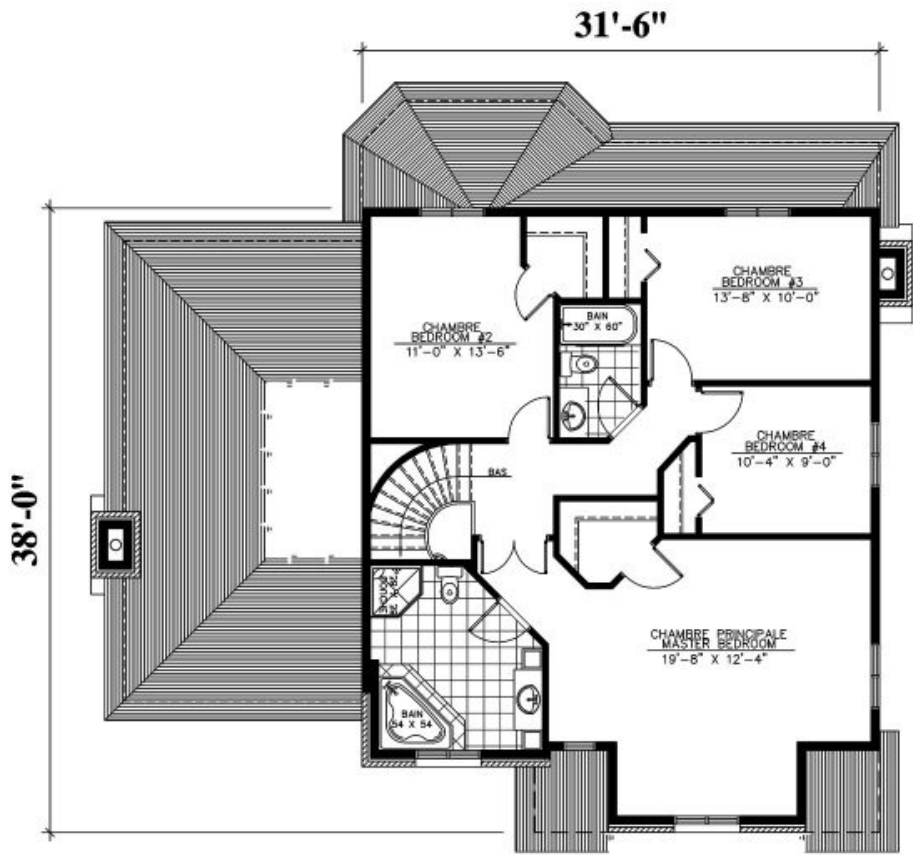
ÉTAGE : 1111 p.c. SECOND FLOOR : 1111 sq.ft.
