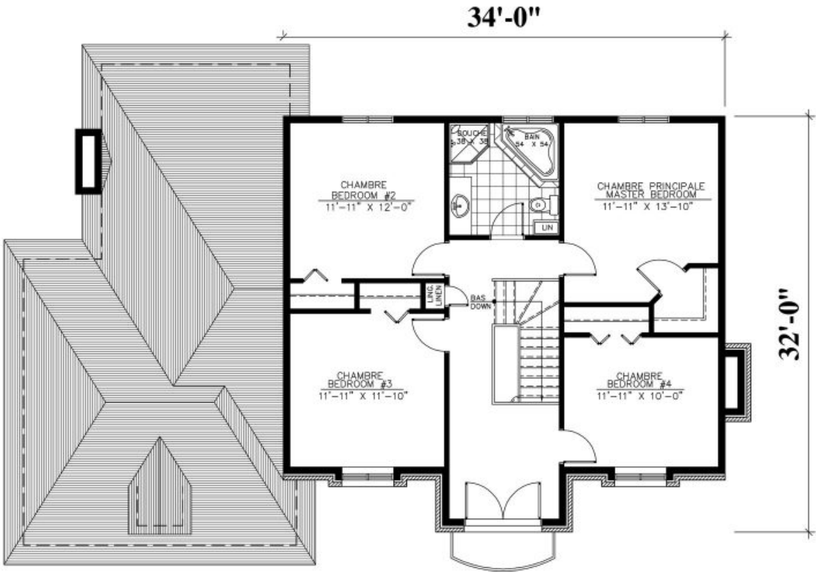
ÉTAGE : 1000 p.c. SECOND FLOOR : 1000 sq.ft.
