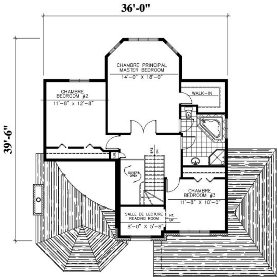
ÉTAGE : 1013 p.c. SECOND FLOOR : 1013 sq.ft.
