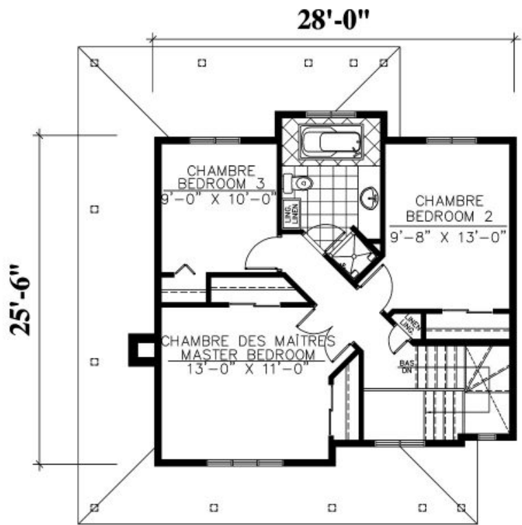
ÉTAGE : 708 p.c. SECOND FLOOR : 708 sq.ft.
