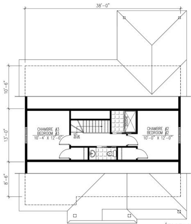
ÉTAGE : 456 p.c. SECOND FLOOR : 456 sq.ft.
