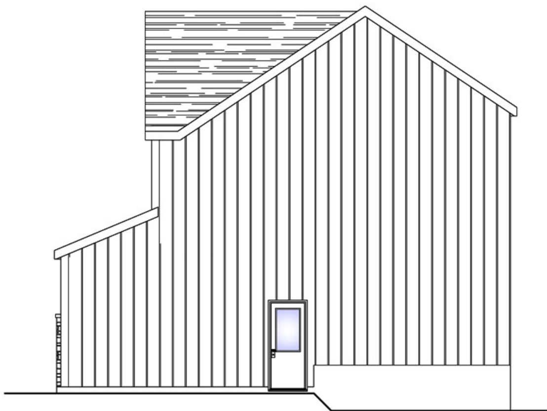
ÉLÉVATION DROITE
