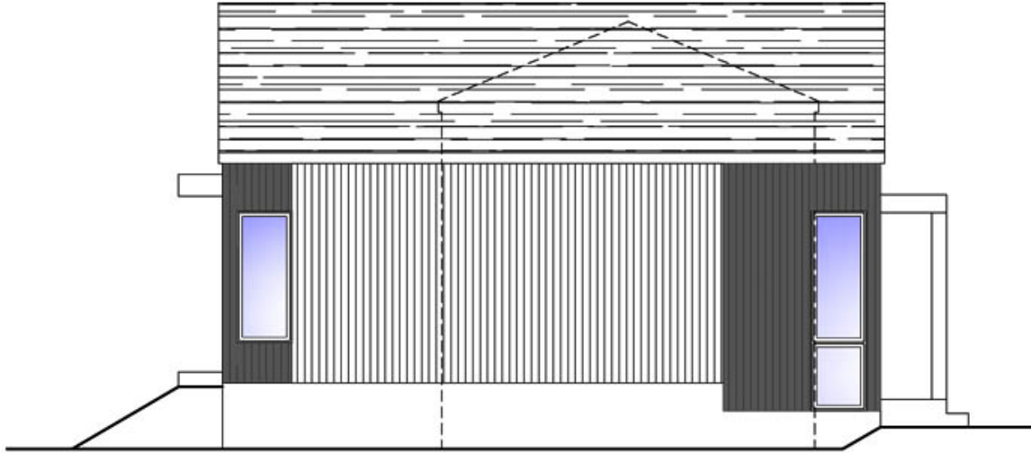
ÉLÉVATION GAUCHE
