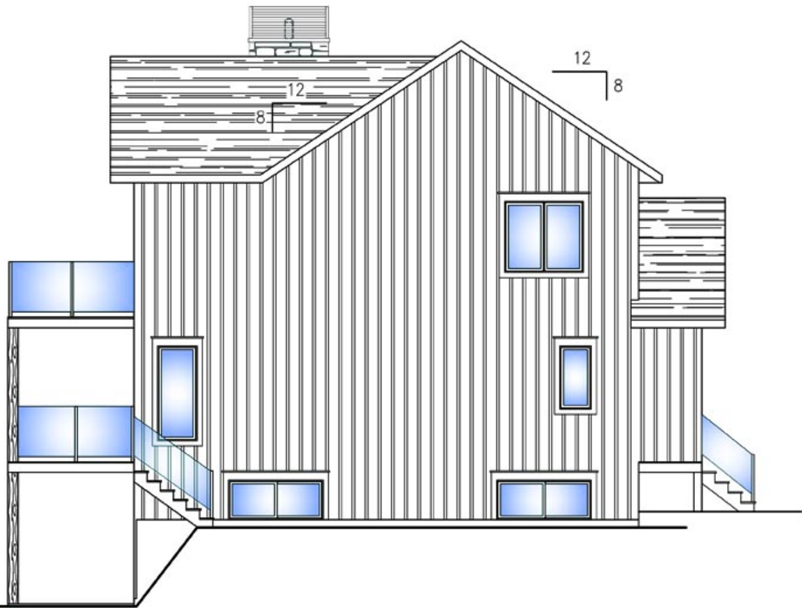
ÉLÉVATION GAUCHE
