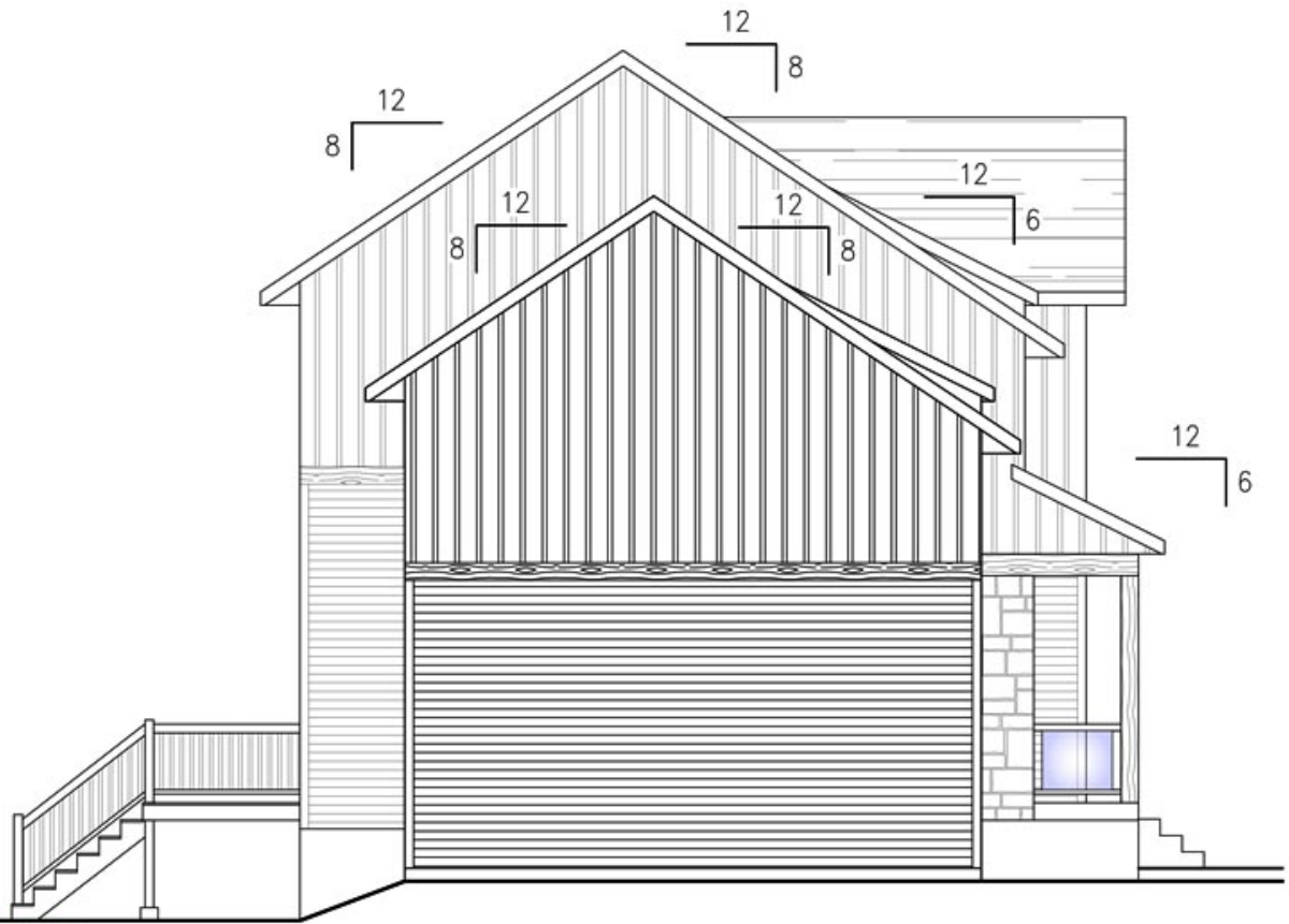
ÉLÉVATION GAUCHE
