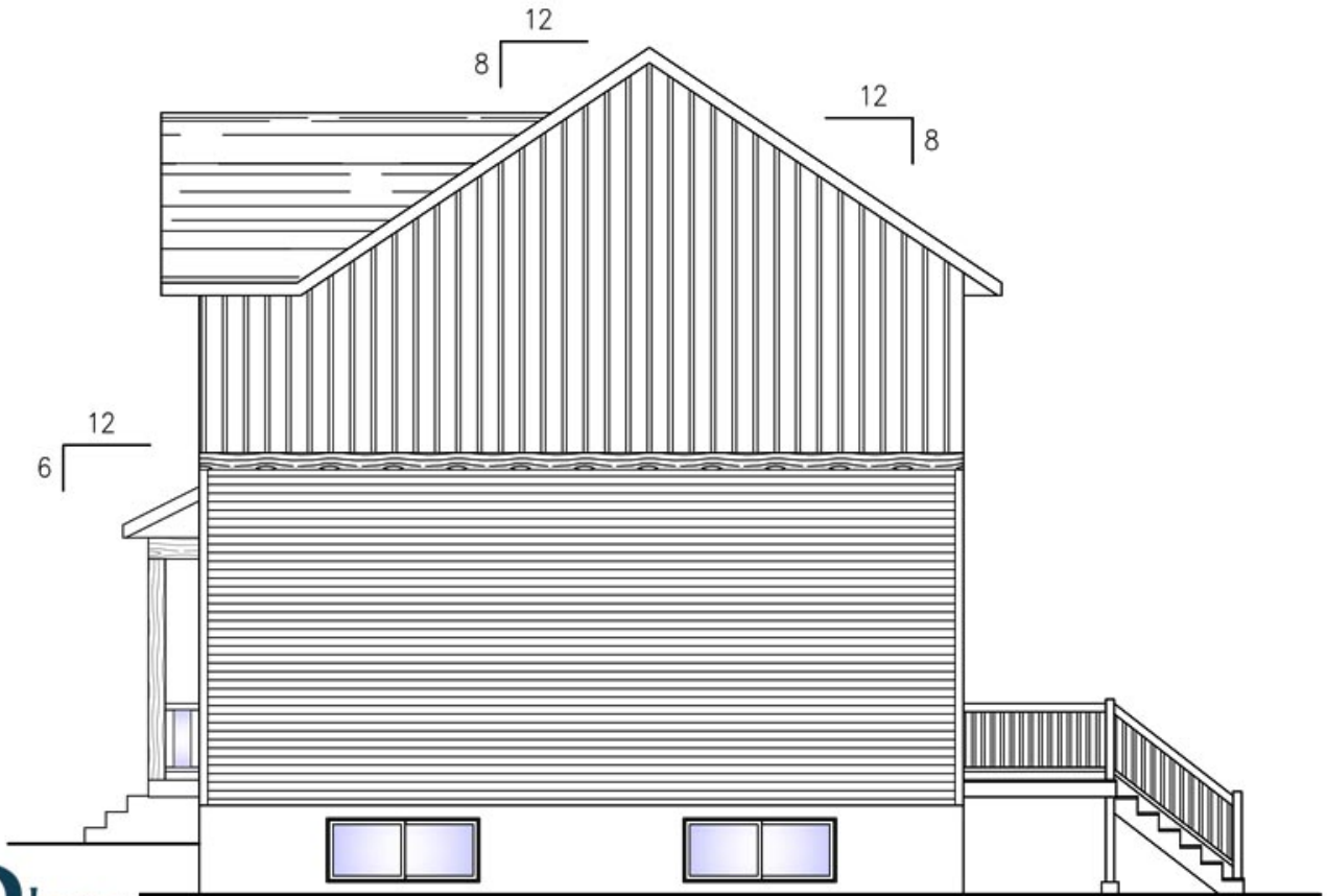
ÉLEVATION DROITE
